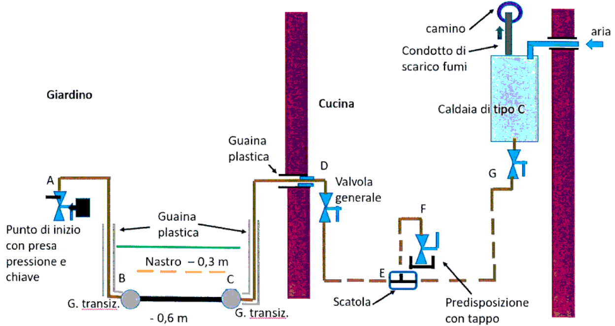
Esempio di schema/elaborato grafico di impianto gas nuovo
